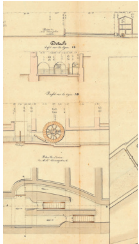
Fig. 43. Bédarieux (Hérault), détail des deux roues hydrauliques de l'usine d'Alexandre Vernazobres ; extrait d'un plan dressé en 1839. © Archives départementales de l'Hérault (France), 7 S 159.
